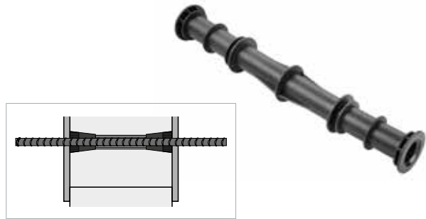
Mod. Tubo rápido encofrado - pasamuro Fast formwork tube Tuyau de passage rapide de coffrage
