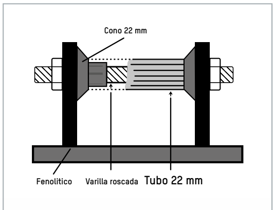
Mod. Tubo encofrado - pasamuro Ø 22 Formwork tube Ø 22 Tuyau de passage de coffrage Ø 22
