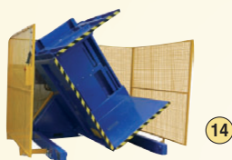
Ref. 5032 INCLINADOR DE CONTENEDORES DE 20°
