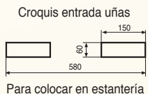
Ref. 3058 Para bidones de 200 lts de chapa Dimensiones (L x A x H) 1.700 x 1.025 x 700 mm Carga 400 kg • Peso 75 kg Radio de giro 90°
